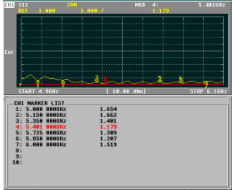
V.S.W.R
